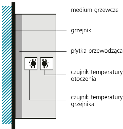
Rys. 2. Schemat budowy elektronicznego podzielnika kosztów ogrzewania, dwuczujnikowego
