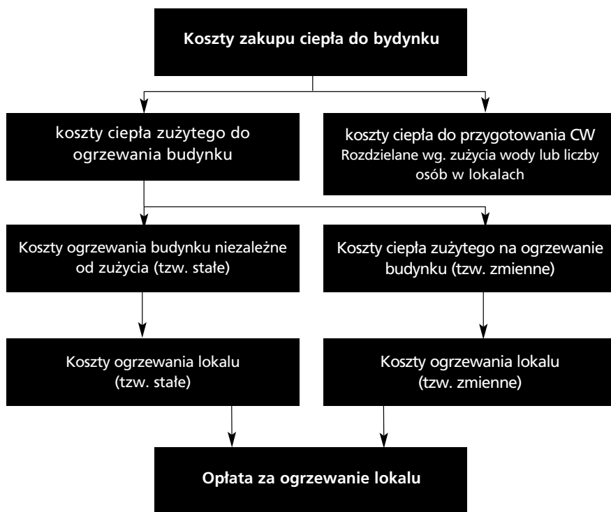
Rys. 3. Schemat rozliczenia kosztów ciepła w budynku według indywidualnego zużycia.
