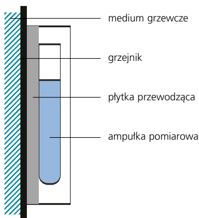
Rys. 1. Schemat budowy cieczowego podzielnika kosztów ogrzewania
